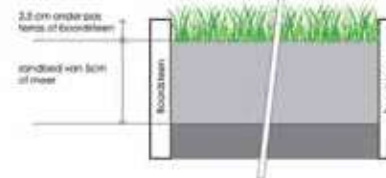
Doorsnede opbouw ondergrond tuin Grasslook®
